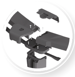
STRUCTURE SUPÉRIEURE
